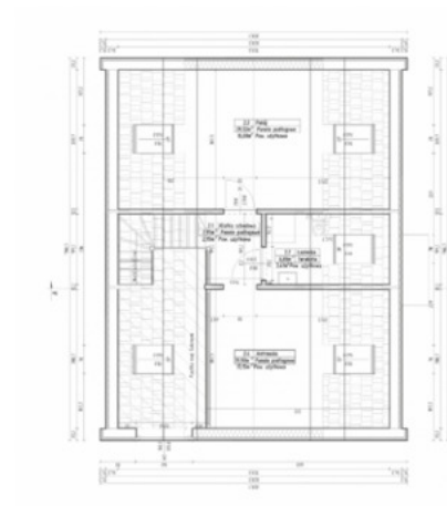
RZUT PODDASZA (ANTRESOLA)
